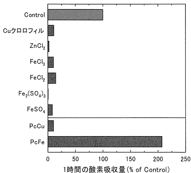
図3 触媒の種類の検討
