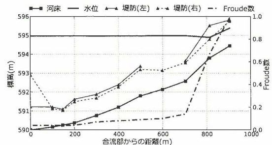
図10 保谷沢川の推定結果（水位とFroude数）
