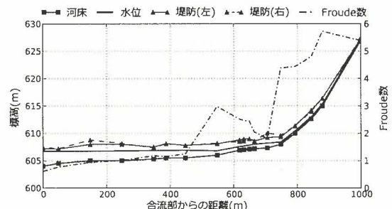
図6 猪の沢川の推定結果（水位とFroude数）
