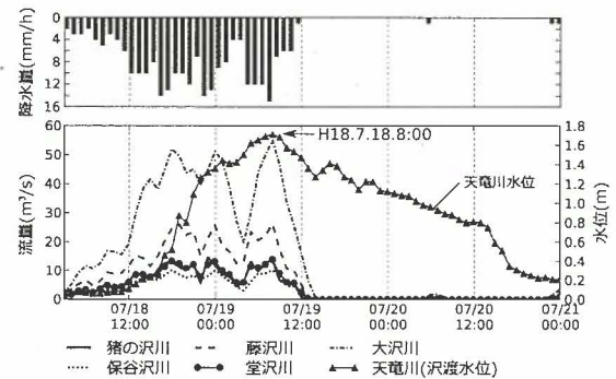
図4 H18.7豪雨時の降雨量（AMeDAS）と天竜川観測水位（沢渡水位観測所），ならびに支流からの推定ハイドログラフ
