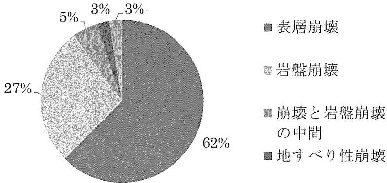
図一四 地震によって発生した斜面崩壊箇所の形態の割合 (n=40)
