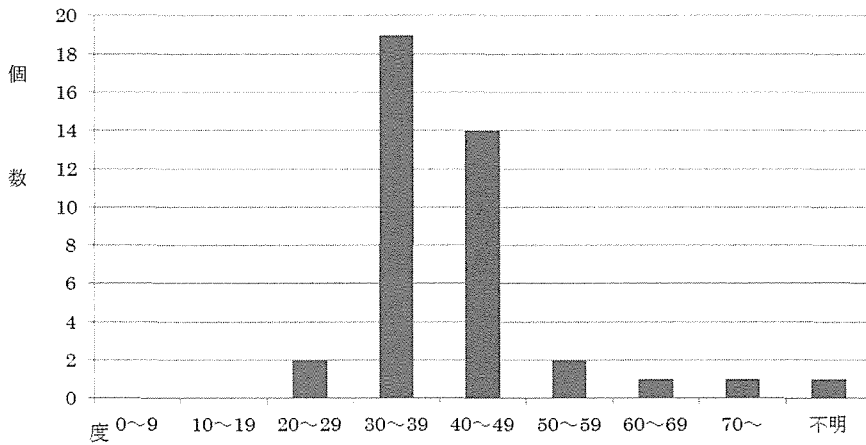
図一五 地震によって発生した斜面崩壊箇所の勾配 (n=40)
