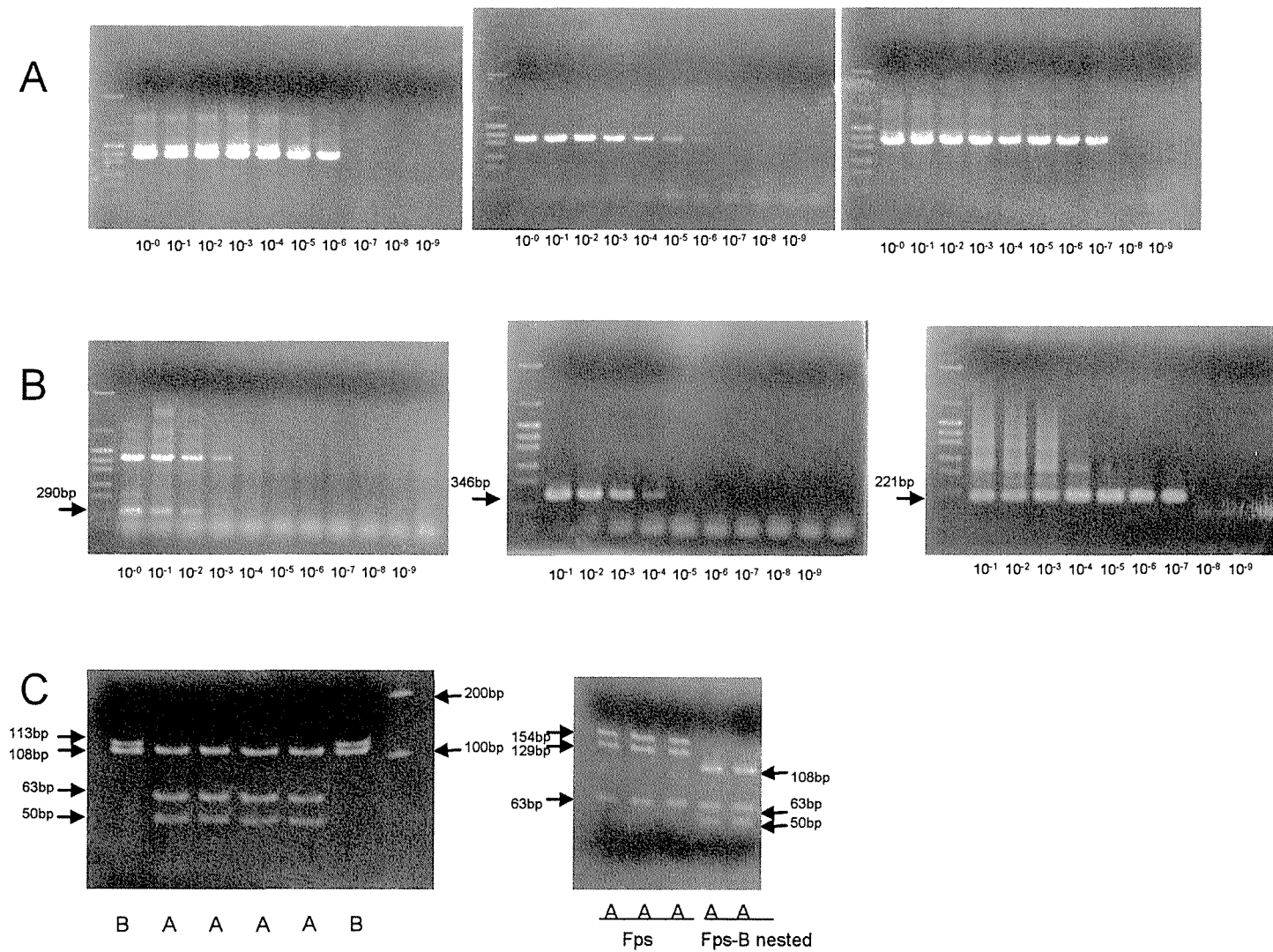
第1図 冷水病菌検出PCRの比較.
