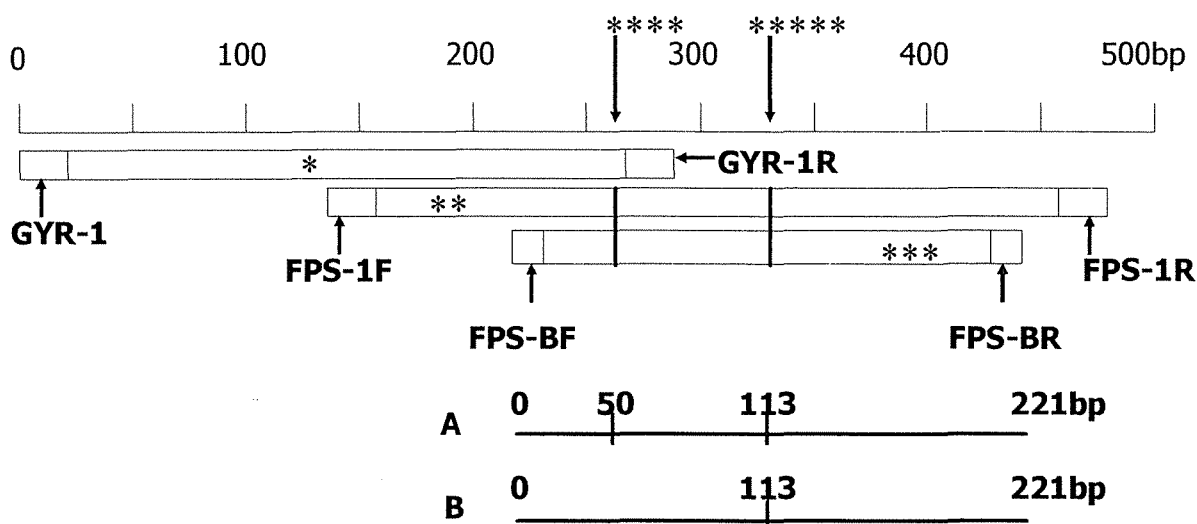
第2図 冷水病菌のA, B遺伝子型を決めるロタマゼ遺伝子領域の検出に用いる3種類のプライマーセットの位置関係
