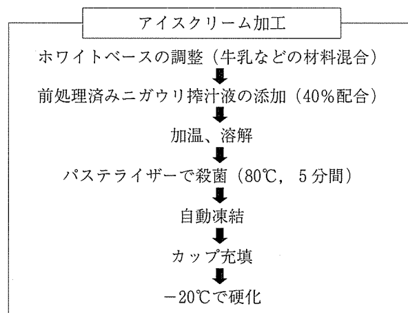
図1 ニガウリアイスクリームの製造工程
