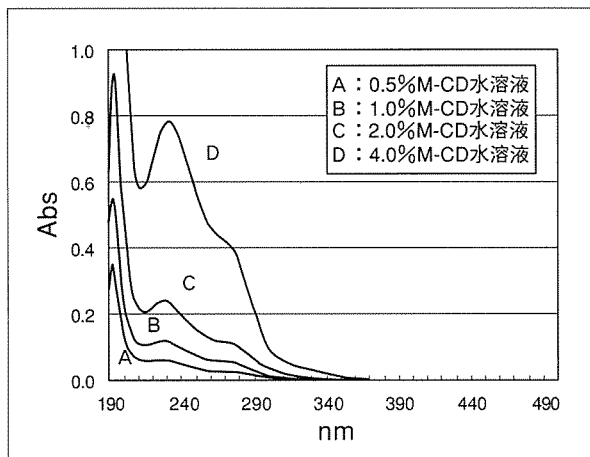
図2 種々のM-CD濃度におけるククルピタシンEの吸収スペクトル
