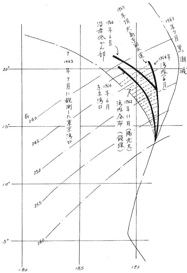
才1図 湾内水塊組成の模式図
