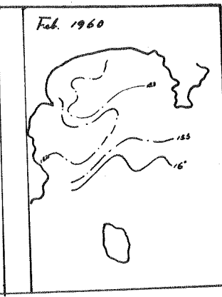
才5図 湾内暖水舌張り出しの例
