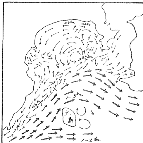
才2図 冬季相模湾総合的潮流図 (宇田:水産試験場報告才8号)
