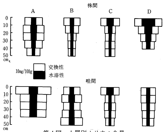
第4図 土層別カリウム含量
