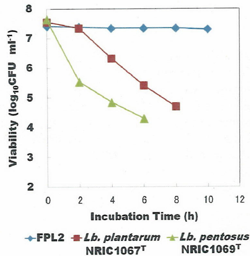
第3図 FPL2と近縁株との耐酸性の比較 *CFUは Colony forming units の略
