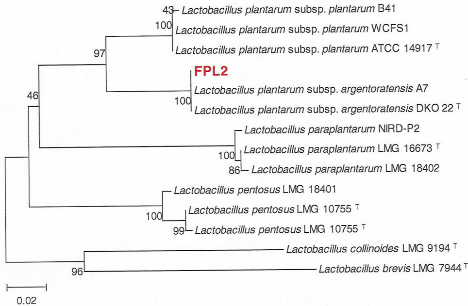
第1図 FPL2のrecA遺伝子塩基配列に基づく分子系統樹
