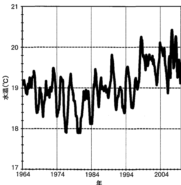
図2 山口県萩市沖における表層水温(12ヶ月移動平均値)の経年変化
